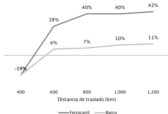
Gráfica 2.6 Ahorro potencial promedio por ferrocarril y barco respecto al autotransporte, 2011
