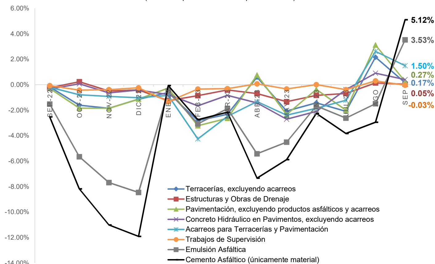
Gráfica 5 | Variación anualizada en los trabajos de infraestructura carretera (Periodo septiembre 2022 a septiembre 2023)
