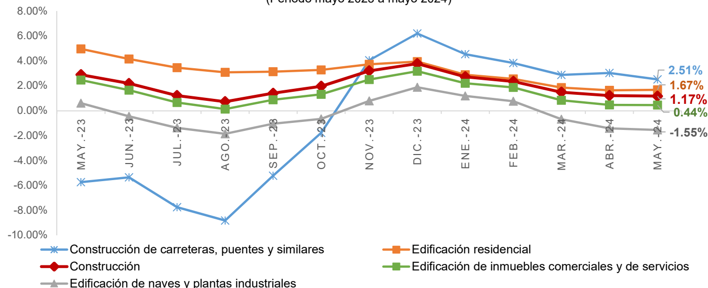
Gráfica 4 | Variación anualizada en el precio de las actividades en el sector de la construcción
