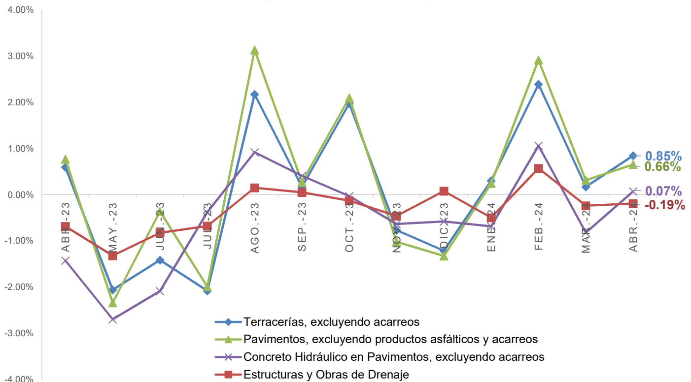
Gráfica 5 | Variación anualizada en los trabajos de infraestructura carretera (Periodo abril 2023 a abril 2024)
