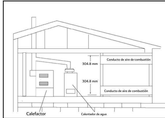
Figura 3303.2 (3) Aparatos ubicados en espacios confinados – todo el aire tomado del exterior a través de un desván
