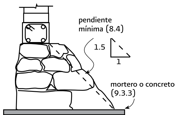
Figura 8.1 Cimiento de piedra
