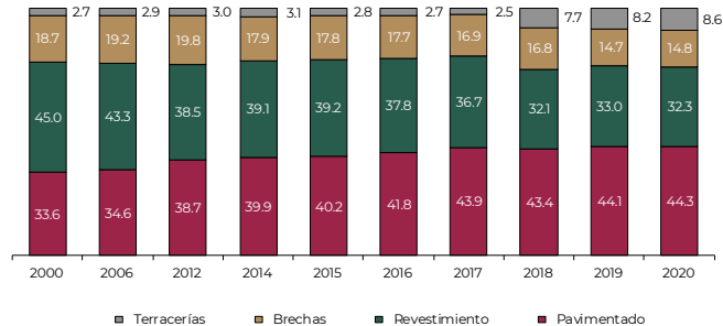
Composición porcentual de la longitud de la red nacional carretera por estado superficial Serie anual 2000, 2006, 2012 y de 2014 a 2020 (Porcentaje)
