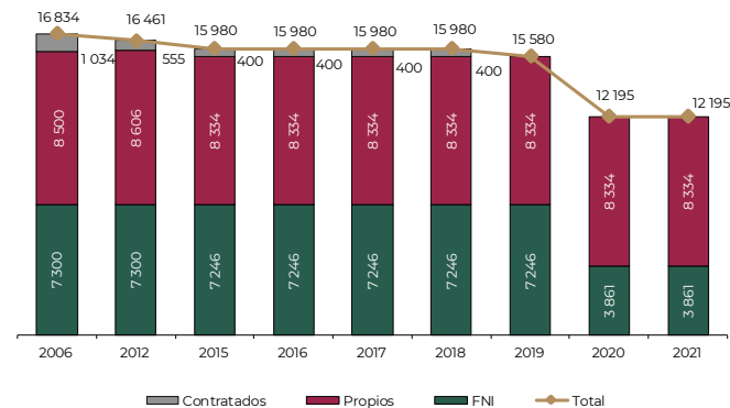
Longitud de la red de puentes de cuota a cargo de CAPUFE por tipo de red Serie anual 2006, 2012, y de 2015 a 2021 (Metros)
