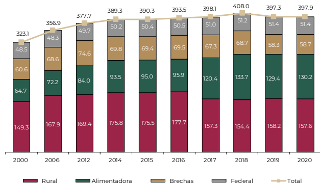
Longitud de la red nacional carretera por tipo de red Serie anual 2000, 2006, 2012 y de 2014 a 2020 (Miles de kilómetros)
